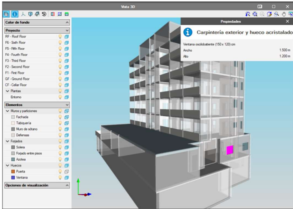
Visualización 3D en IFC Builder (CYPE)
