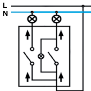
Interruptor doble con indicador luminoso WL024X
