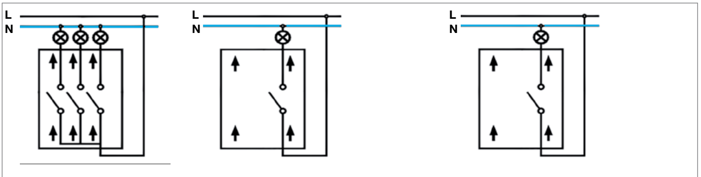
Interrupor con indicador luminoso WL021X
