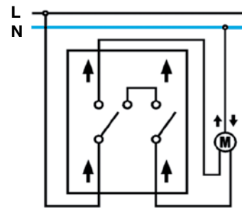
Interruptor para persiana WL031X
