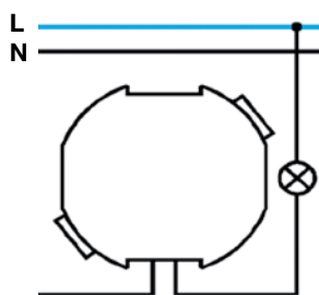
Regulador rotativo WL401X /403X
