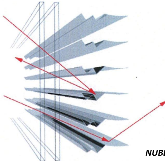
Lichtlenkjalousie
