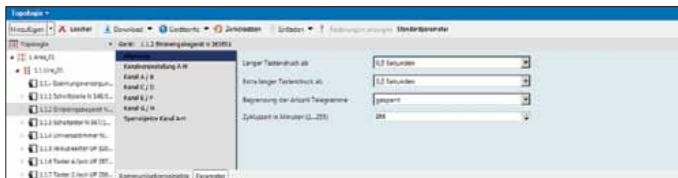
Imagen 32. Definición de parámetros de dispositivos.
