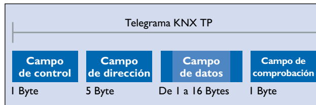
Imagen 7. Estructura de telegrama en KNX TP.
